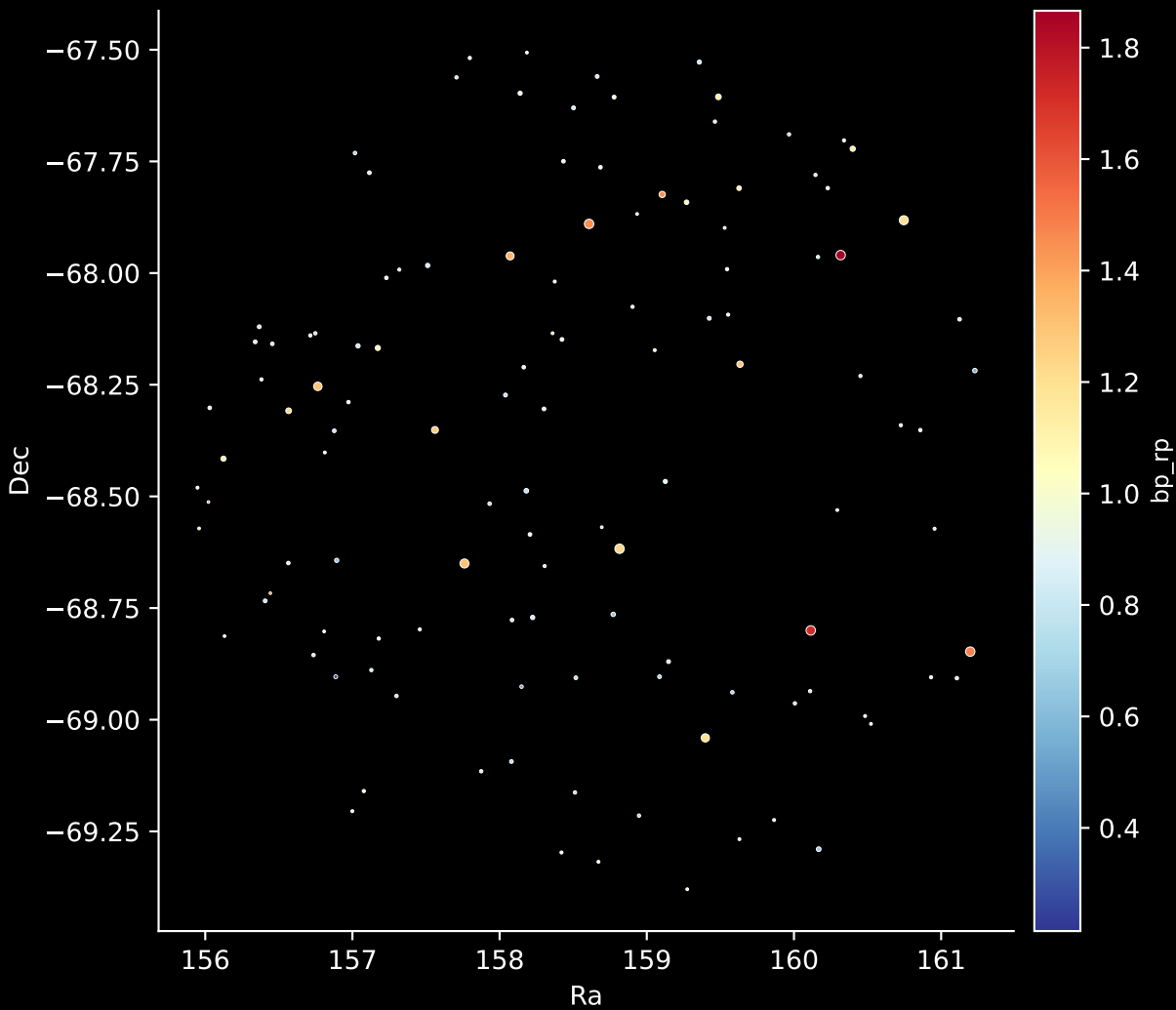
GALAH DR4 Field: [7245] Stars: 119
