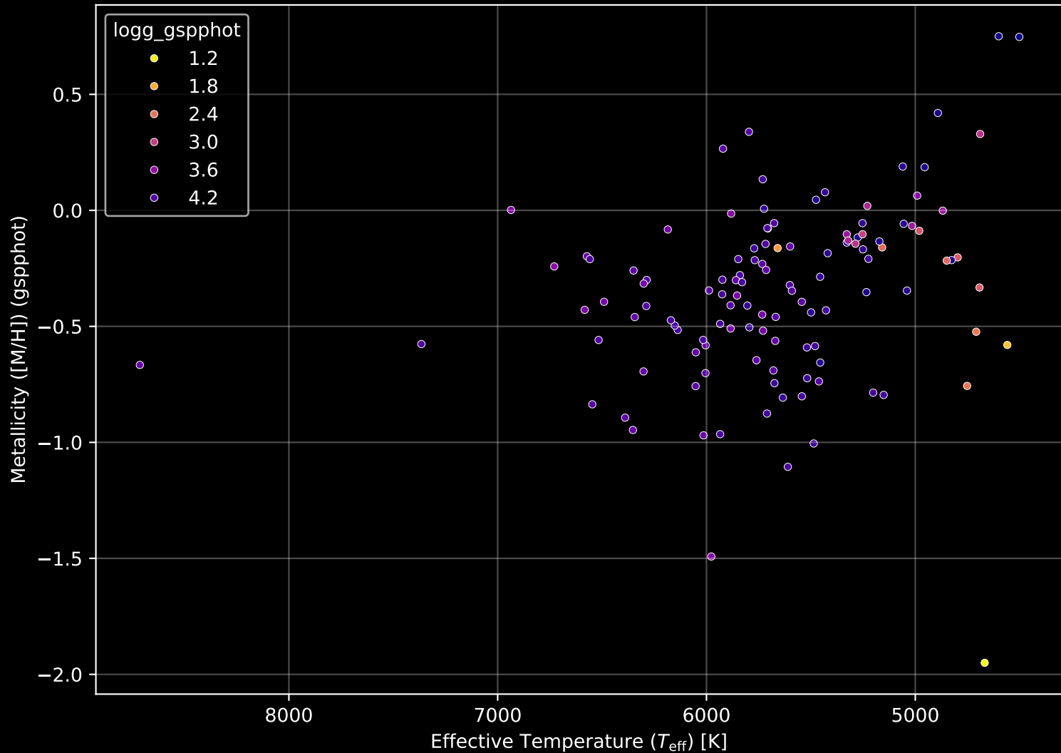
GALAH DR4 Field: [7245] Stellar Population Parameters (n= 119)
